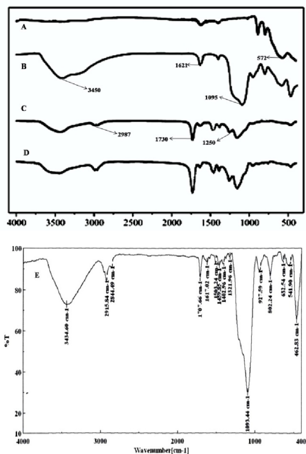
Figure 3. FT-IR spectra of \text{Fe}_3\text{O}_4 (A), \text{Fe}_3\text{O}_4@\text{SiO}_2 (B), \text{Fe}_3\text{O}_4@\text{SiO}_2@\text{MPS} (C), \text{Fe}_3\text{O}_4@\text{NIPs} (D), and \text{Fe}_3\text{O}_4@\text{MIPs} (E).
